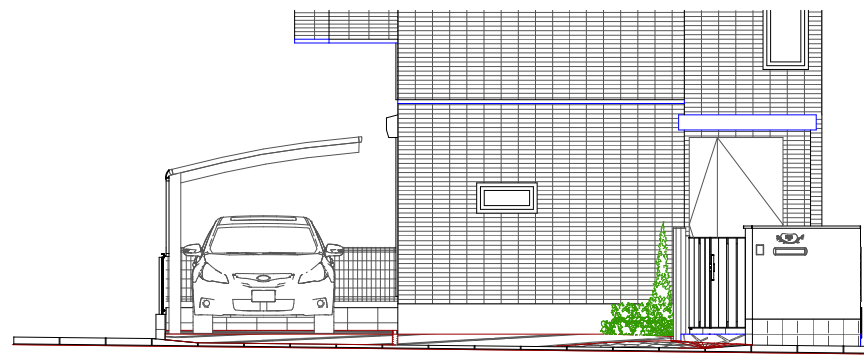
東側立面図
