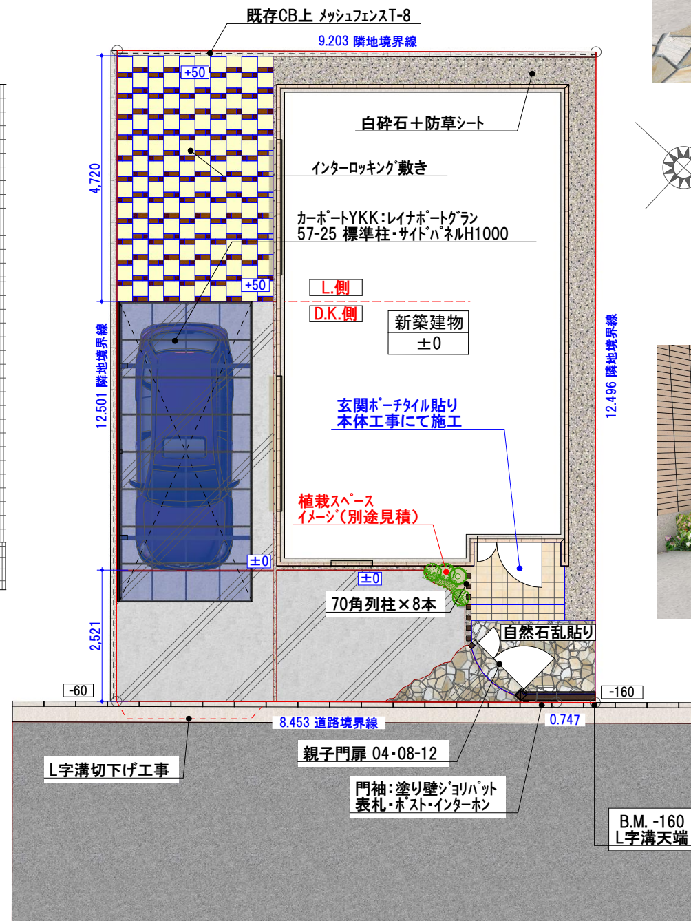
平面図 S: 1/100
