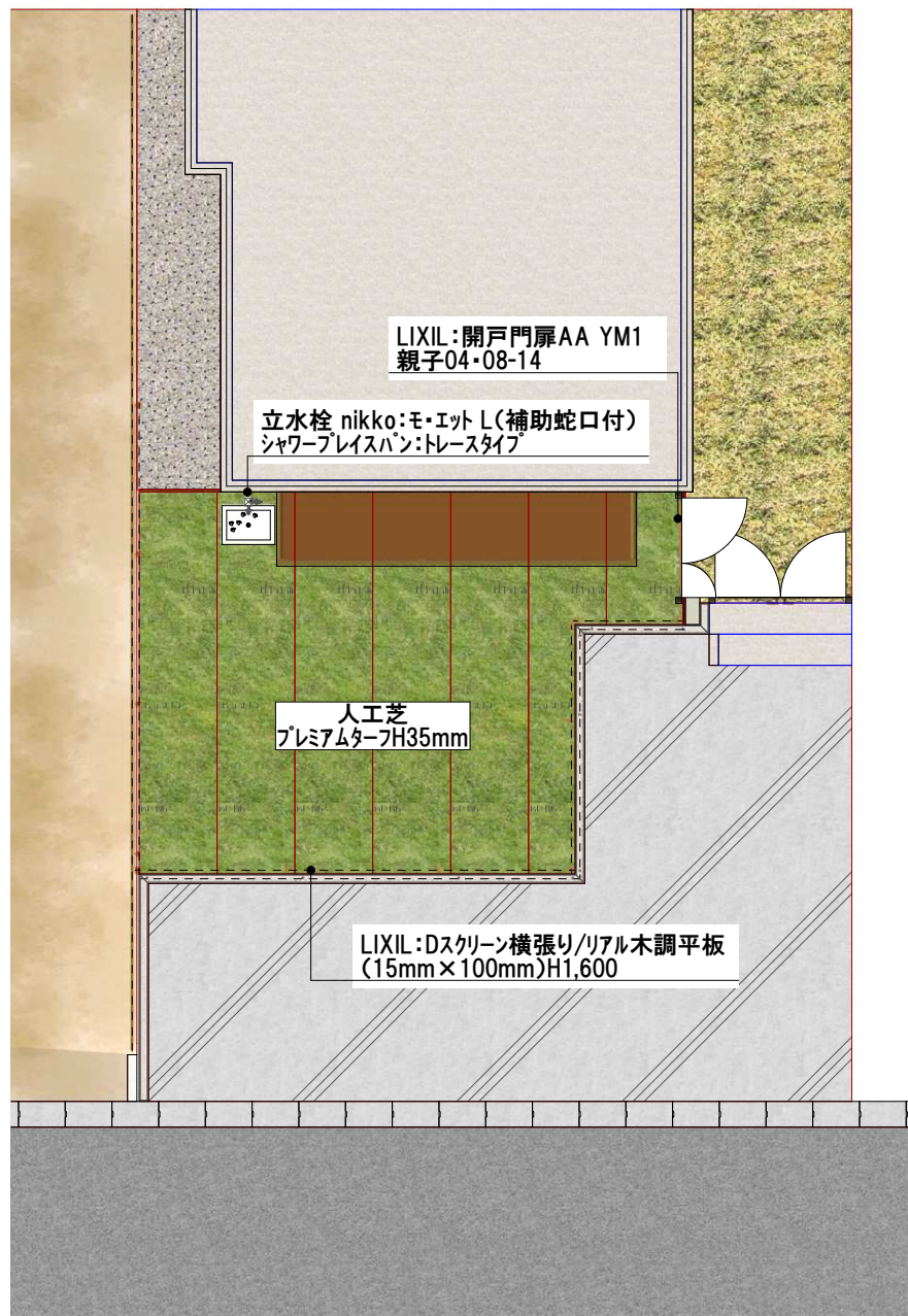
平面図 S:1/100
