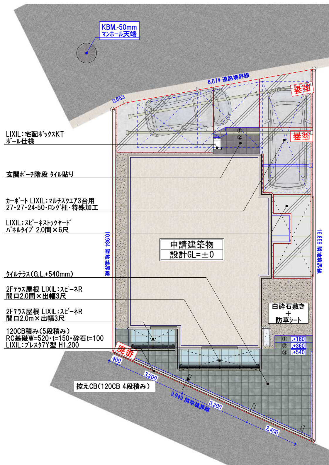
平面図 S:1/100
