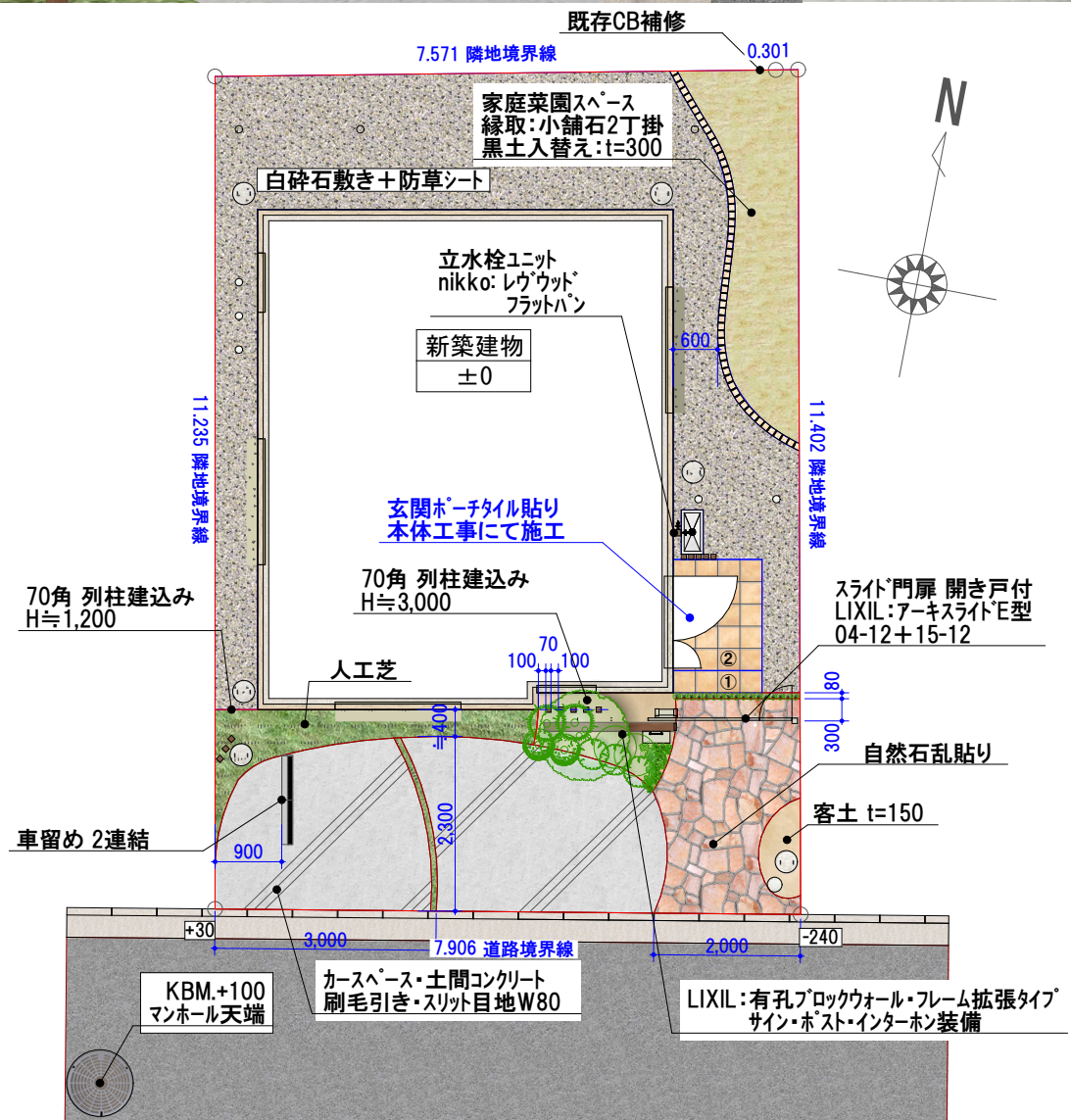
平面図 S:1/100
