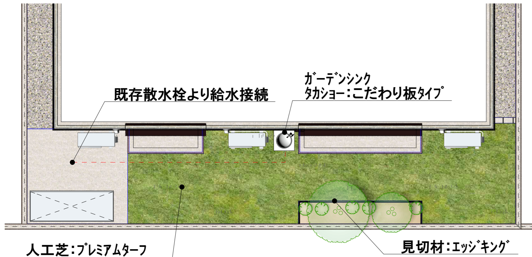
平面図 S:1/50
