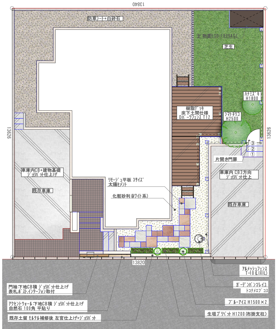
平面図 S:1/100
