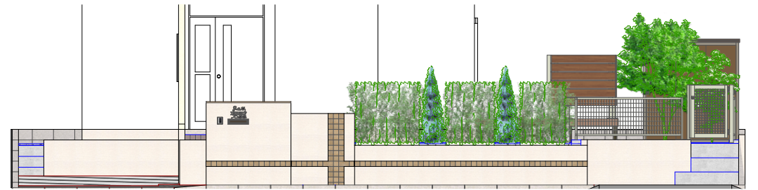
西側立面図
